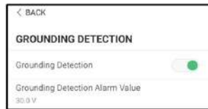
Abbildung 8-40 Erdungskontrolle
